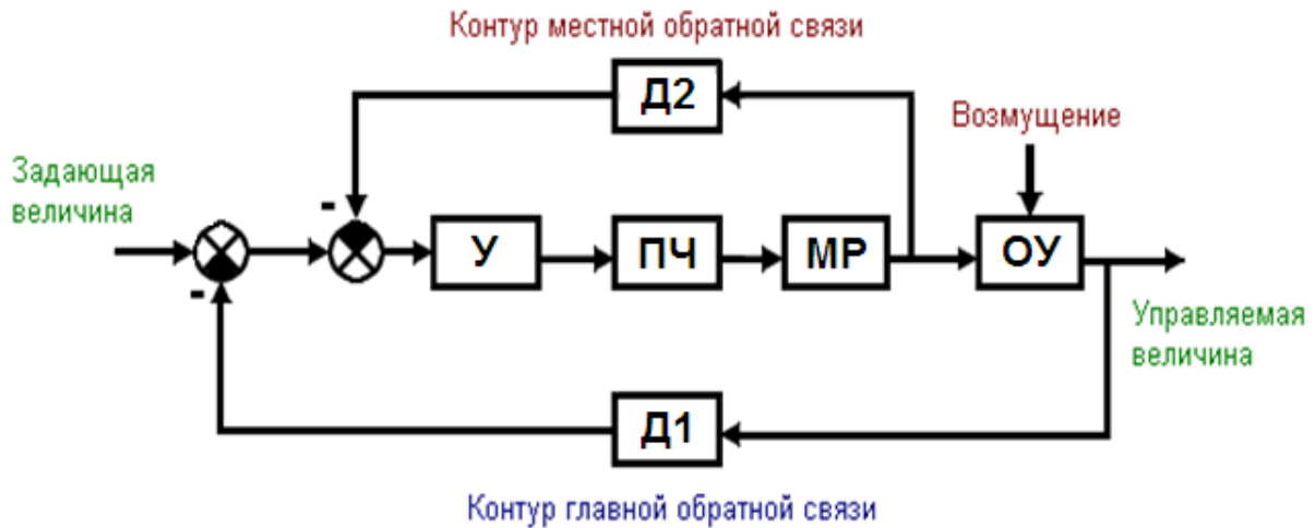
Рисунок 2.1 - Функциональная схема САР
